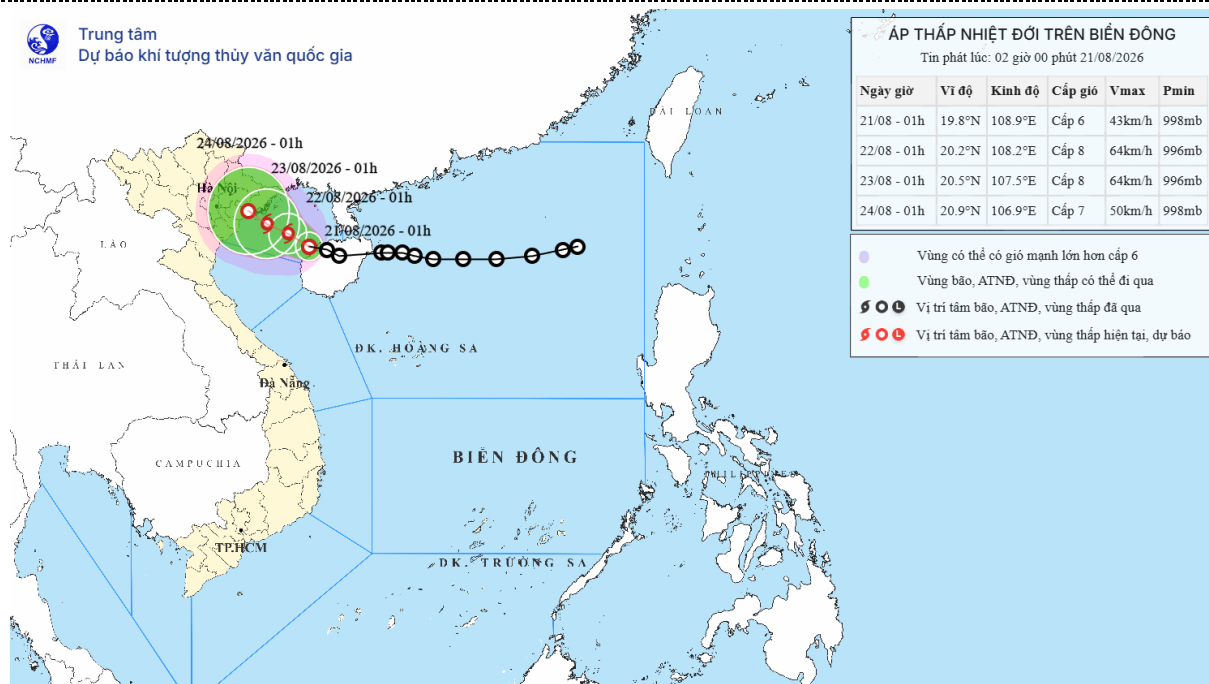
Hình 1. Bản đồ dự báo quỹ đạo và cường độ áp thấp nhiệt đới lúc 02h00 ngày 21/8/2026
